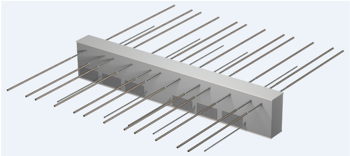
Isopro 80 (Dämmstärke 80 mm)
