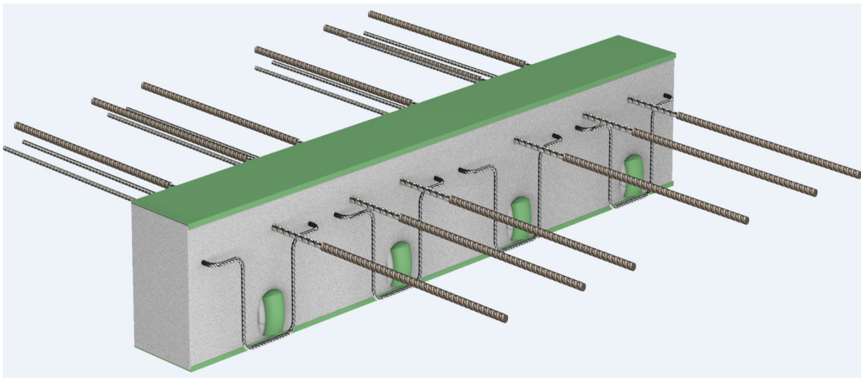
Isopro 120 (Dämmstärke 120 mm)
