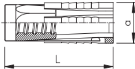
Ausführung 3-schalig (Tragkraft 90 kN)
