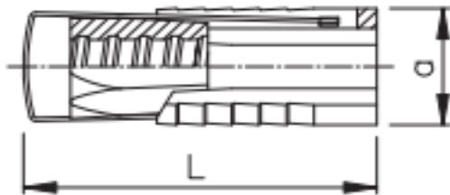
Ausführung 2-schalig (Tragkraft 60 kN)
